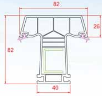
Orta Kayıt
