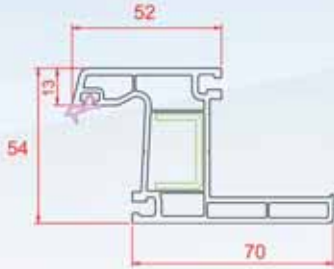
Pervazlı Kasa
