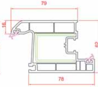
Dar Kapı Kanat
