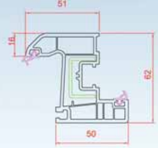
Dar Pencere Kanat
