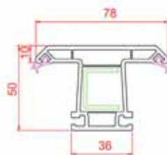
Orta Kayıt
