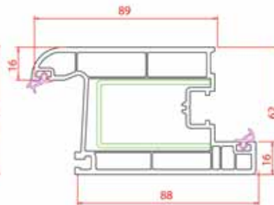
Kapı Kanat
