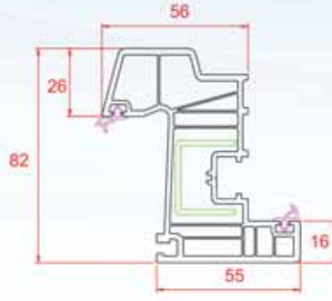
Damlalıklı Kanat
