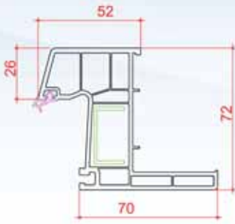
Pervazlı Kasa
