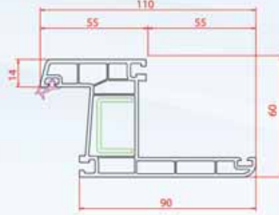
Pervazlı Kasa
