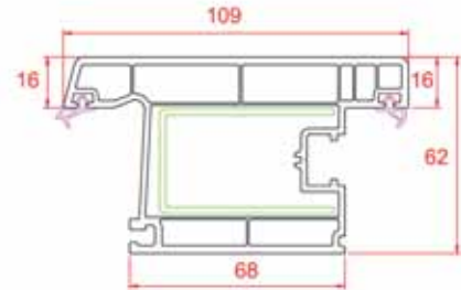
Dışa Açılım Kapı Kanat
