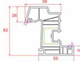
Damlalıklı Kanat
