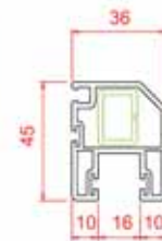
Sineklik
