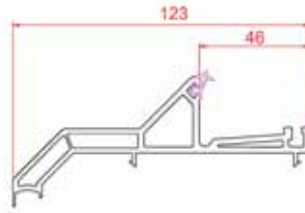
Kasa İçi Orta Kayıt Adaptörü
