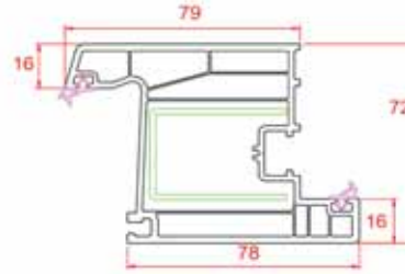
Dar Kapı Kanat
