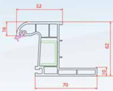
Pervazlı Kasa
