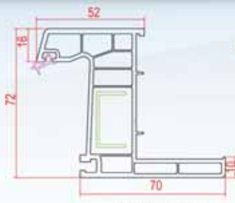
Pervazlı Kasa
