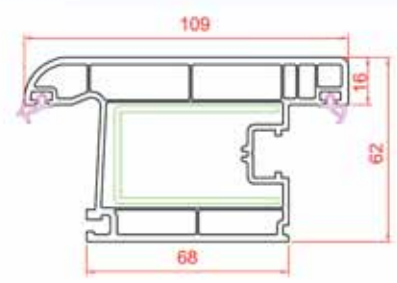
Dışa Açılım Kapı Kanat
