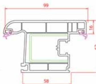
Dar Dış Açılım Kapı Kanat
