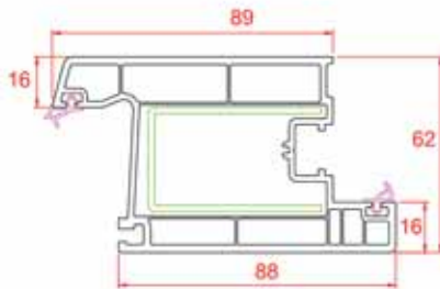
Kapı Kanat
