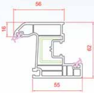
Pencere Kanat
