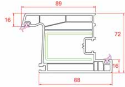
Kapı Kanat
