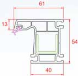
Kasa
