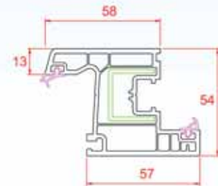
Pencere Kanat
