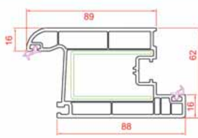
Kapı Kanat
