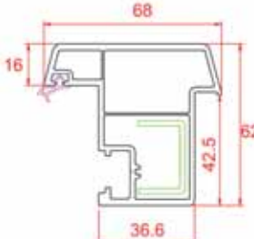
Hareketli Orta Kayıt
