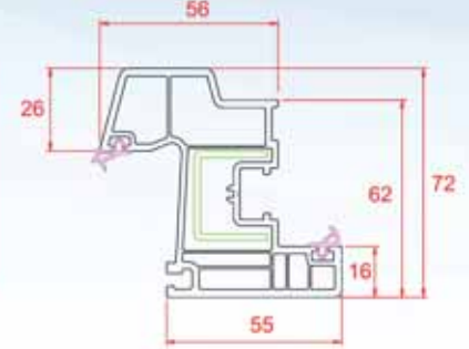
Damlalıklı Kanat
