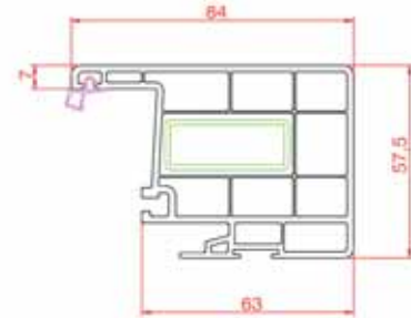
Orta Kayıt
