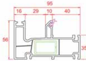
Tekli Kasa
