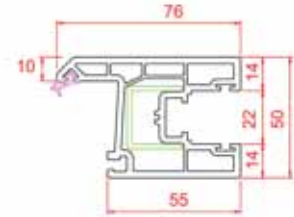
Pencere Kanat
