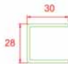
Süper Kasa - Pencere Kanat - Orta Kayıt Destek Sacı
