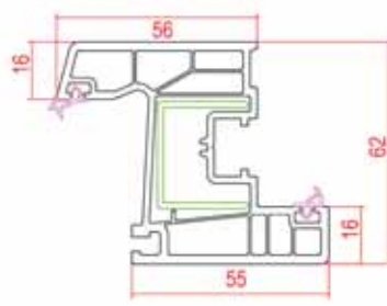
Pencere Kanat
