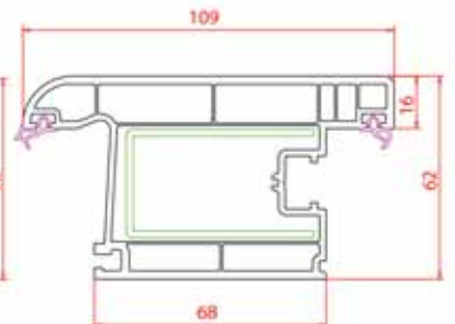
Dış Açılım Kapı Kanat
