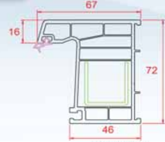
Süper Kasa
