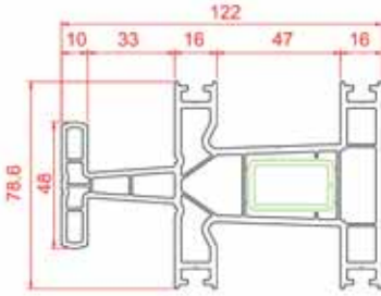
Kasa İçi Orta Kayıt
