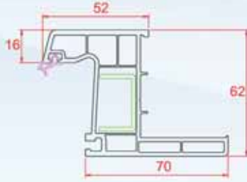
Pervazlı Kasa
